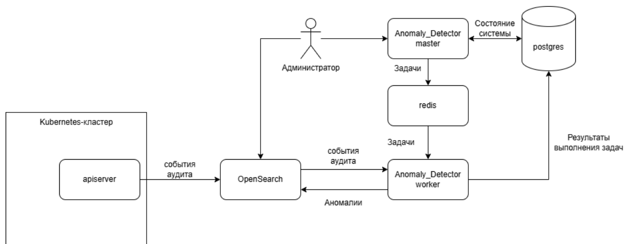
Рисунок 11 – Архитектура программного средства обнаружения аномалий
