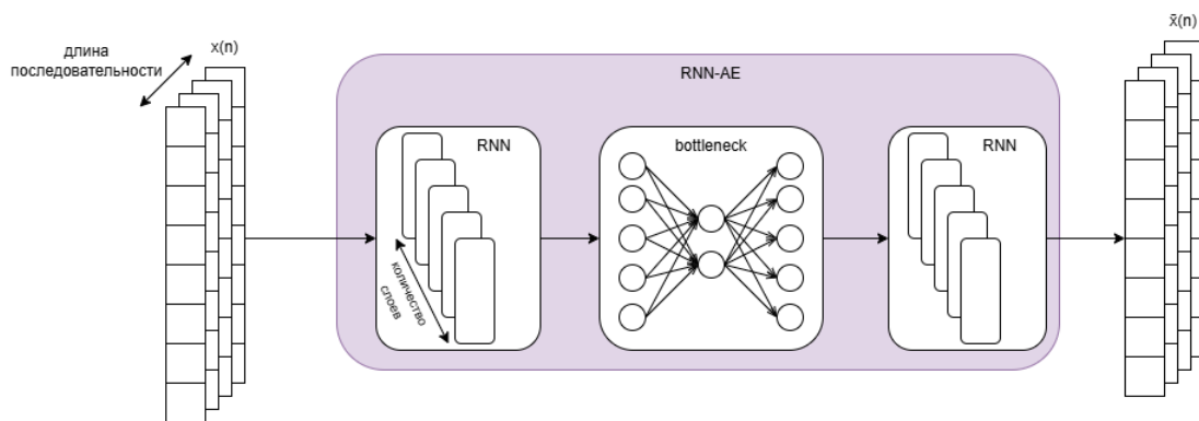
Рисунок 18 – Архитектура RNN-Autoencoder.
